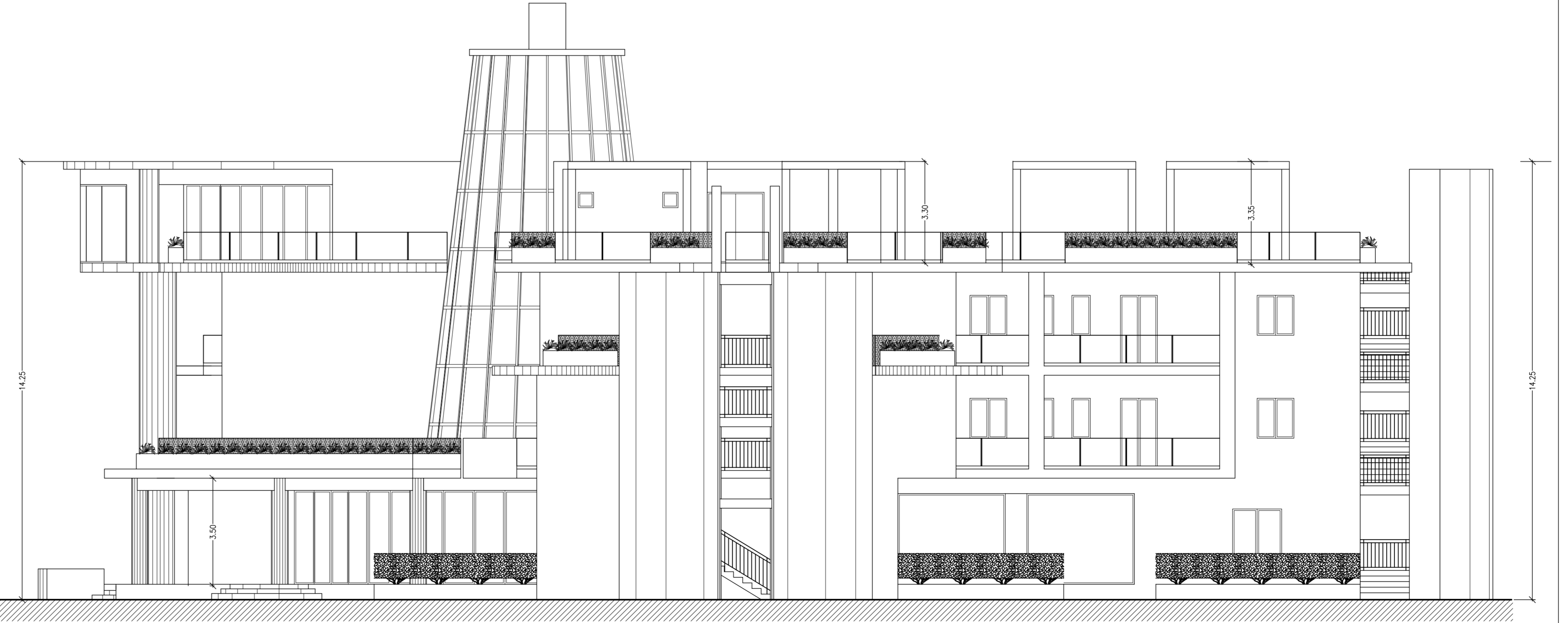
PROSPETTO LATO DESTRO
