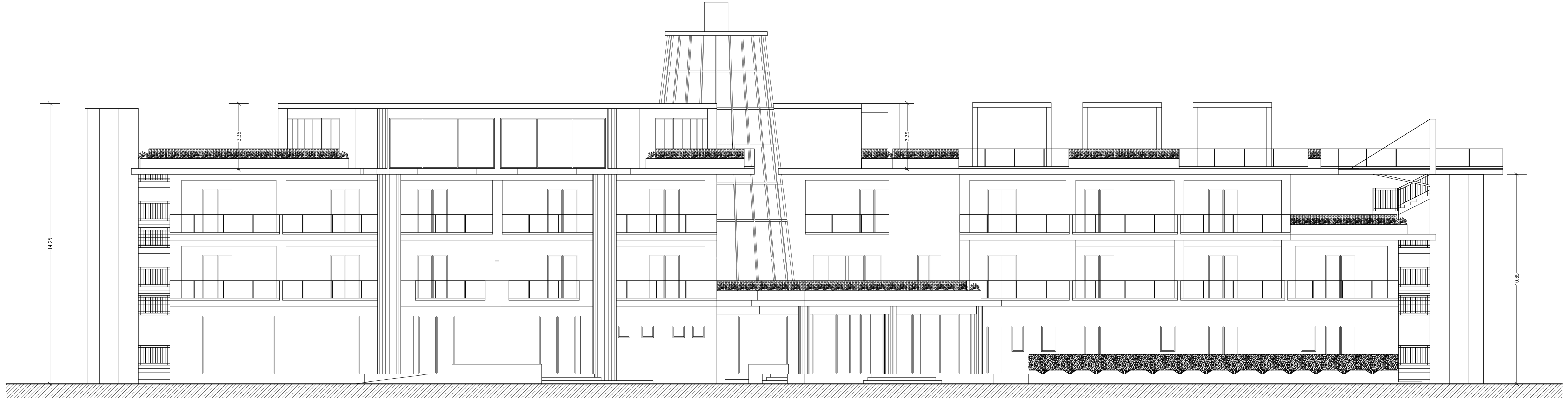
PROSPETTO PRINCIPALE
