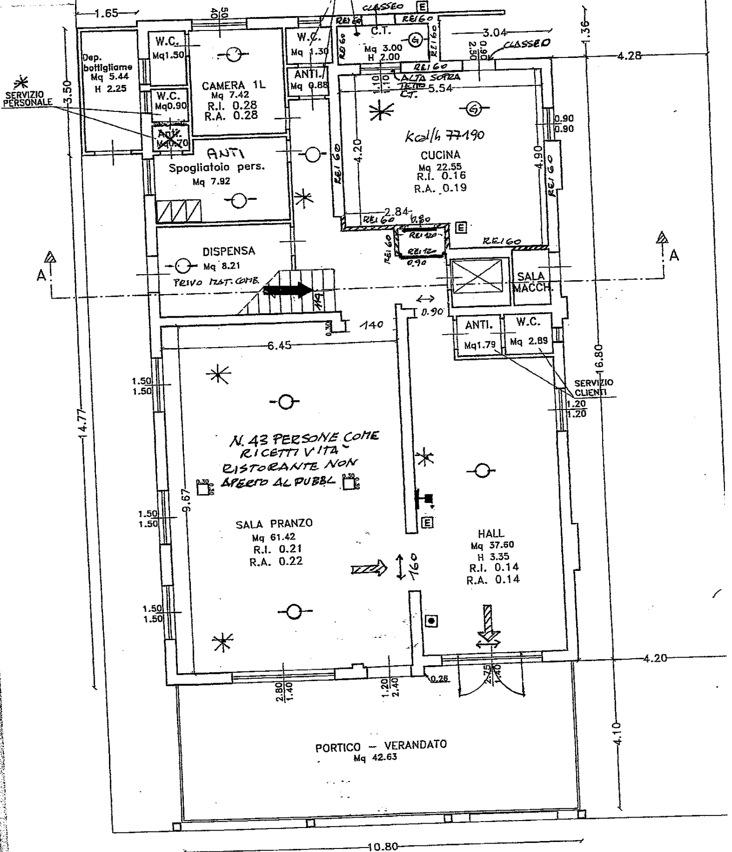
PIANO TERRA H=3.35
